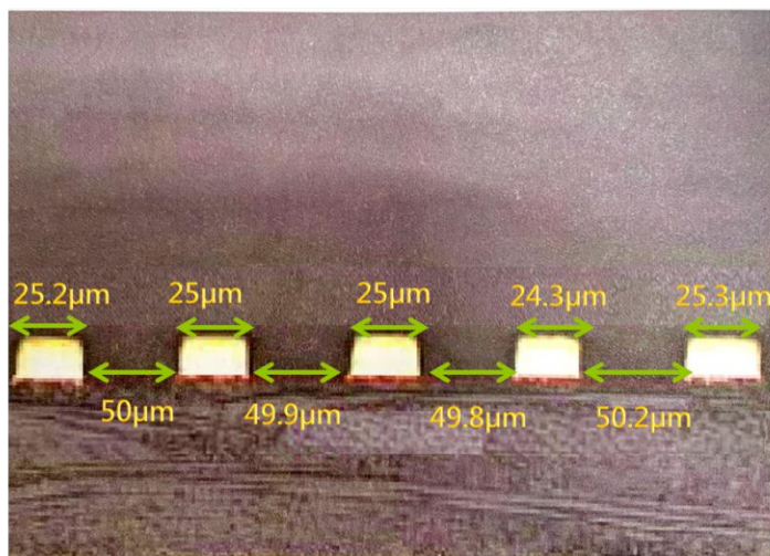
線路蝕刻後剖面圖
