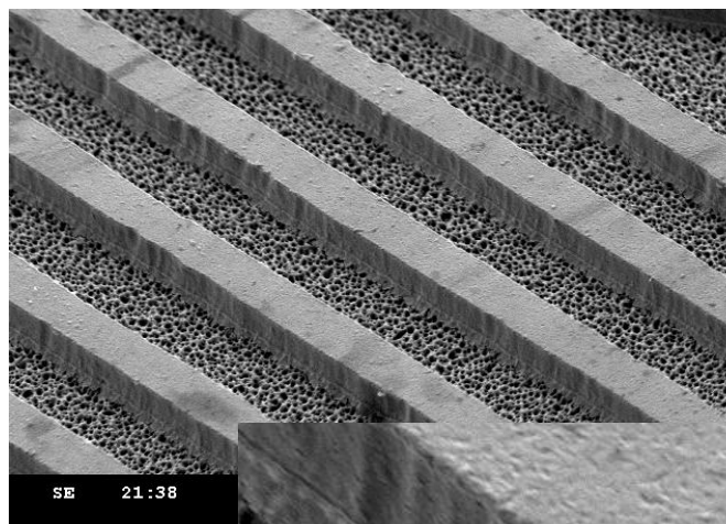
蝕刻後 S E M 圖
