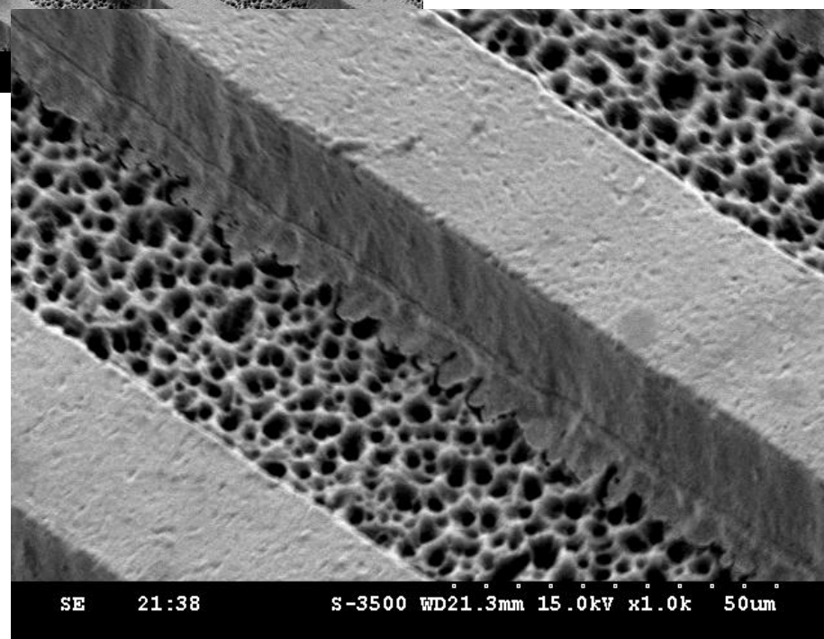
放大後蝕刻後 S E M 圖
